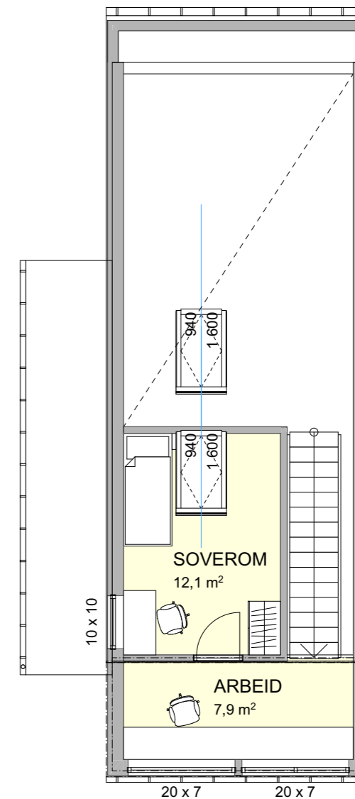
Plan 2.etasje
