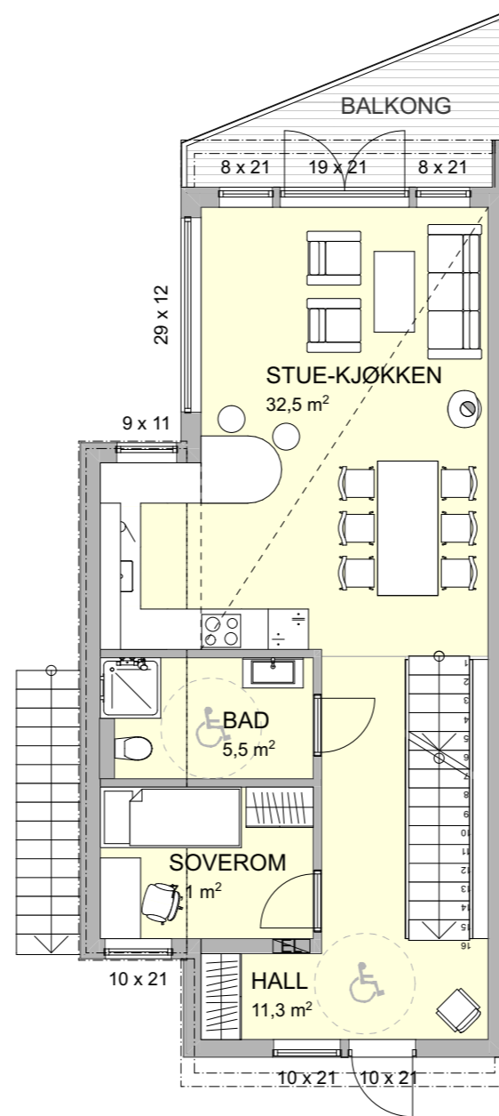
Plan 1.etasje
